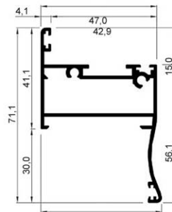
MIT EINEM RUNDEN STIFT TYP B
